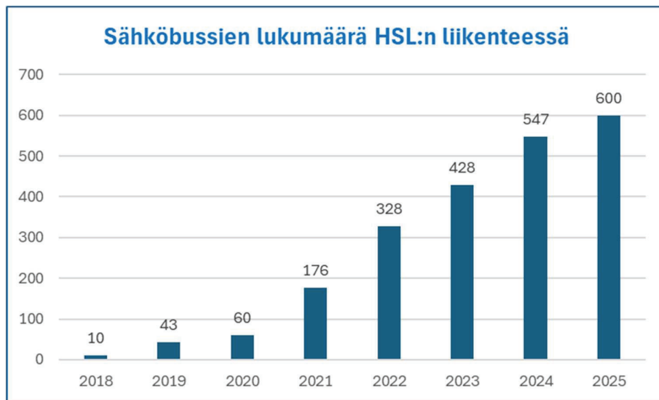
Kuva 4: Sähköbussien määrä 2018-2025
